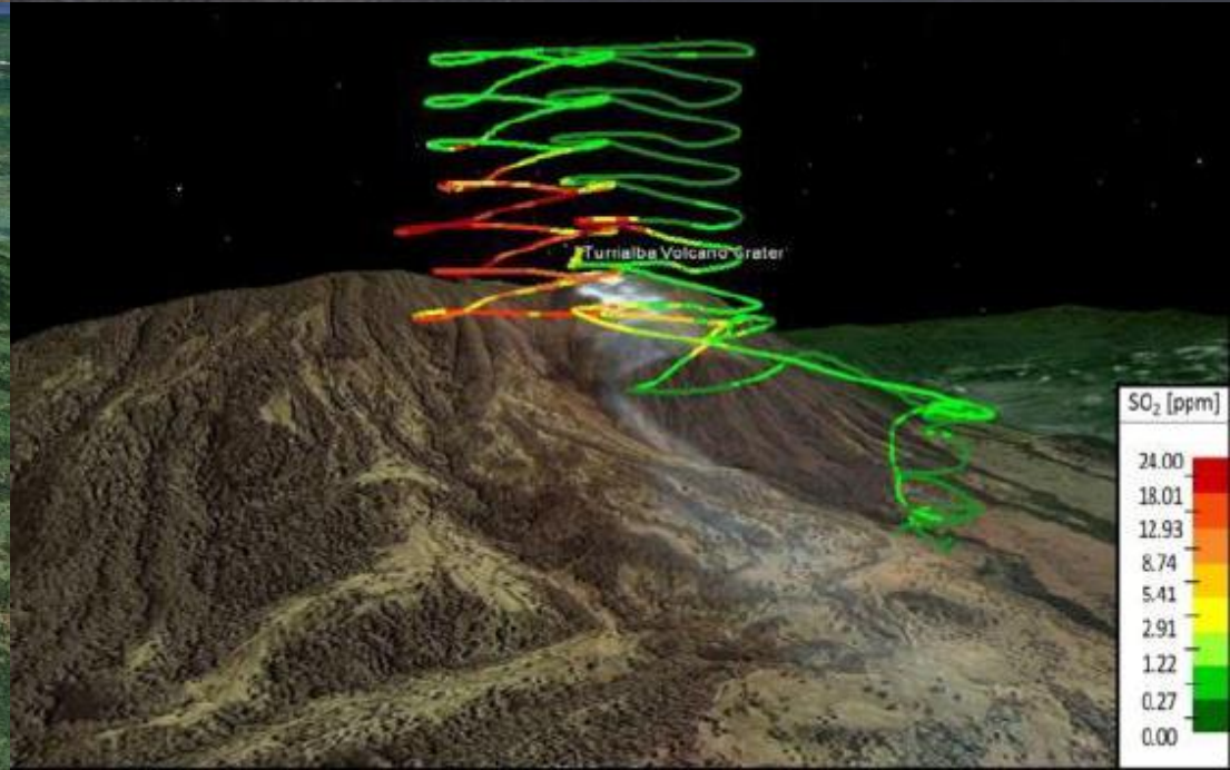
miniGAS GLX on DJI S1000+ UAV Turrialba Volcano.
